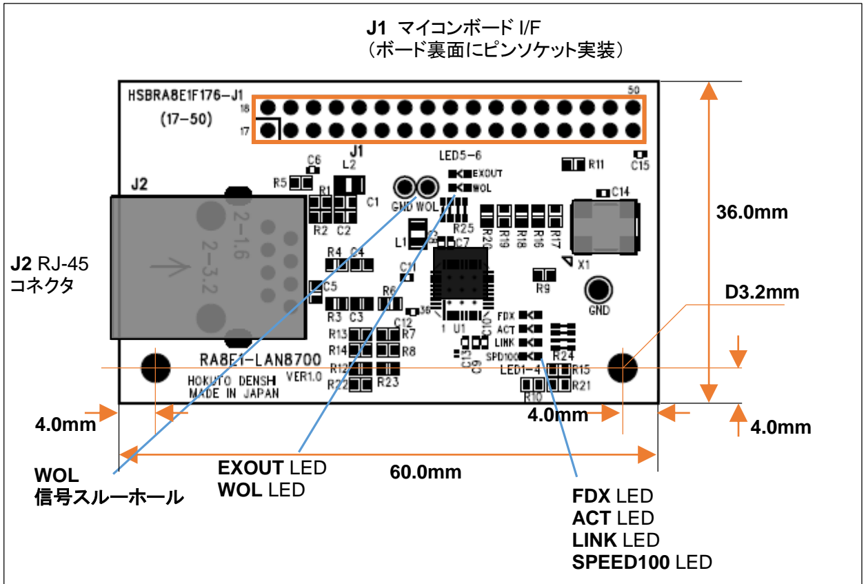
図 1-1 ボード外形(RA8E1-LAN8700)
