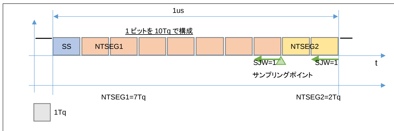
図 5-3 TSEG 固定時の CAN データの 1 ビット
