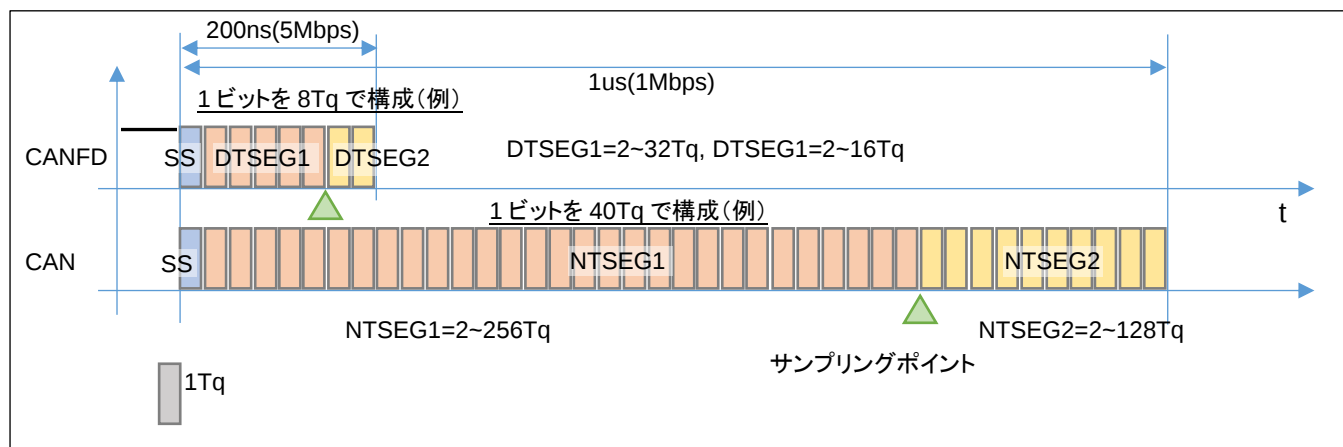
図 5-2 CANFD/CAN データの 1 ビット
