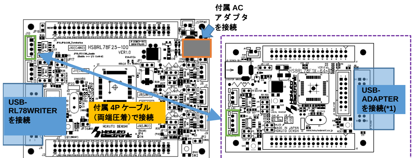
図 1-3 キット接続形態(2)
