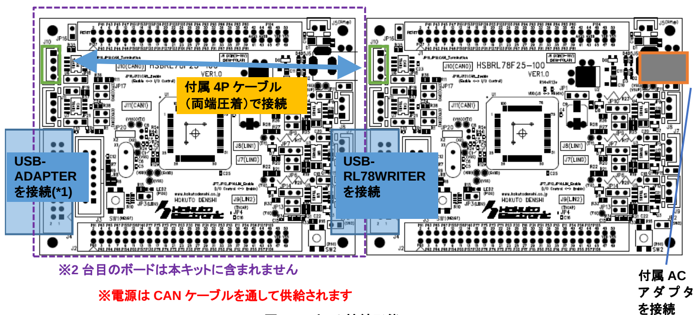
図 1-2 キット接続形態(1)
