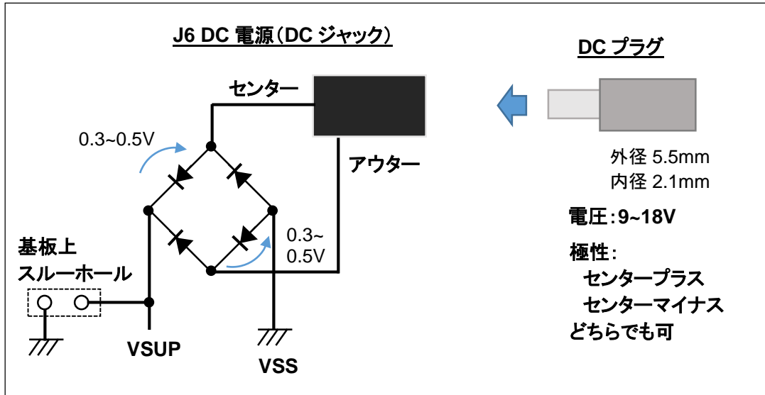
図 2-3 DC ジャック部
