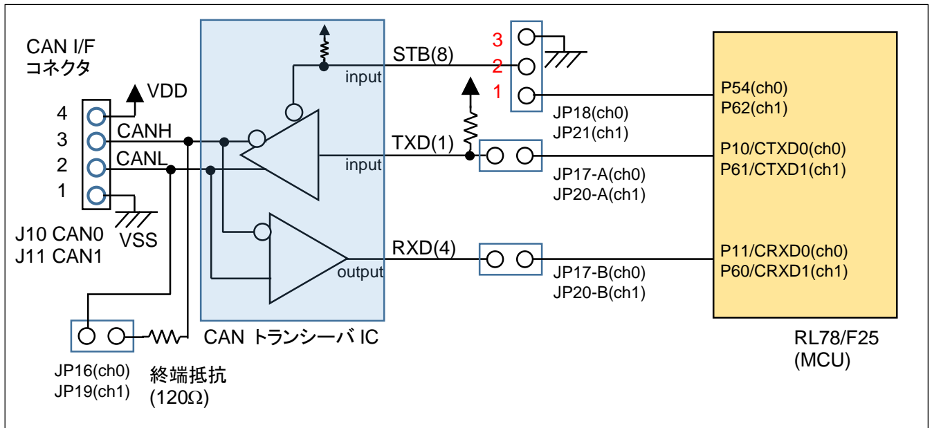
図 2-5 CAN-FD インタフェースブロック図
