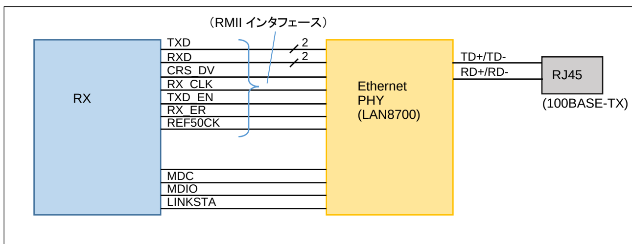
図 1-1b マイコンと LAN コネクタの接続(RMII)
