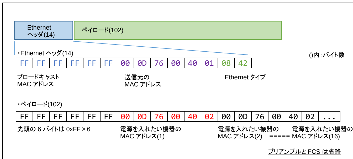
図 3-1 MagicPacket の構造
