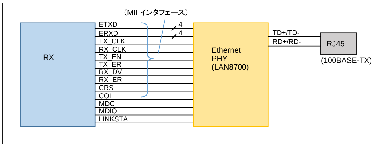
図 1-1a マイコンと LAN コネクタの接続(MII)
