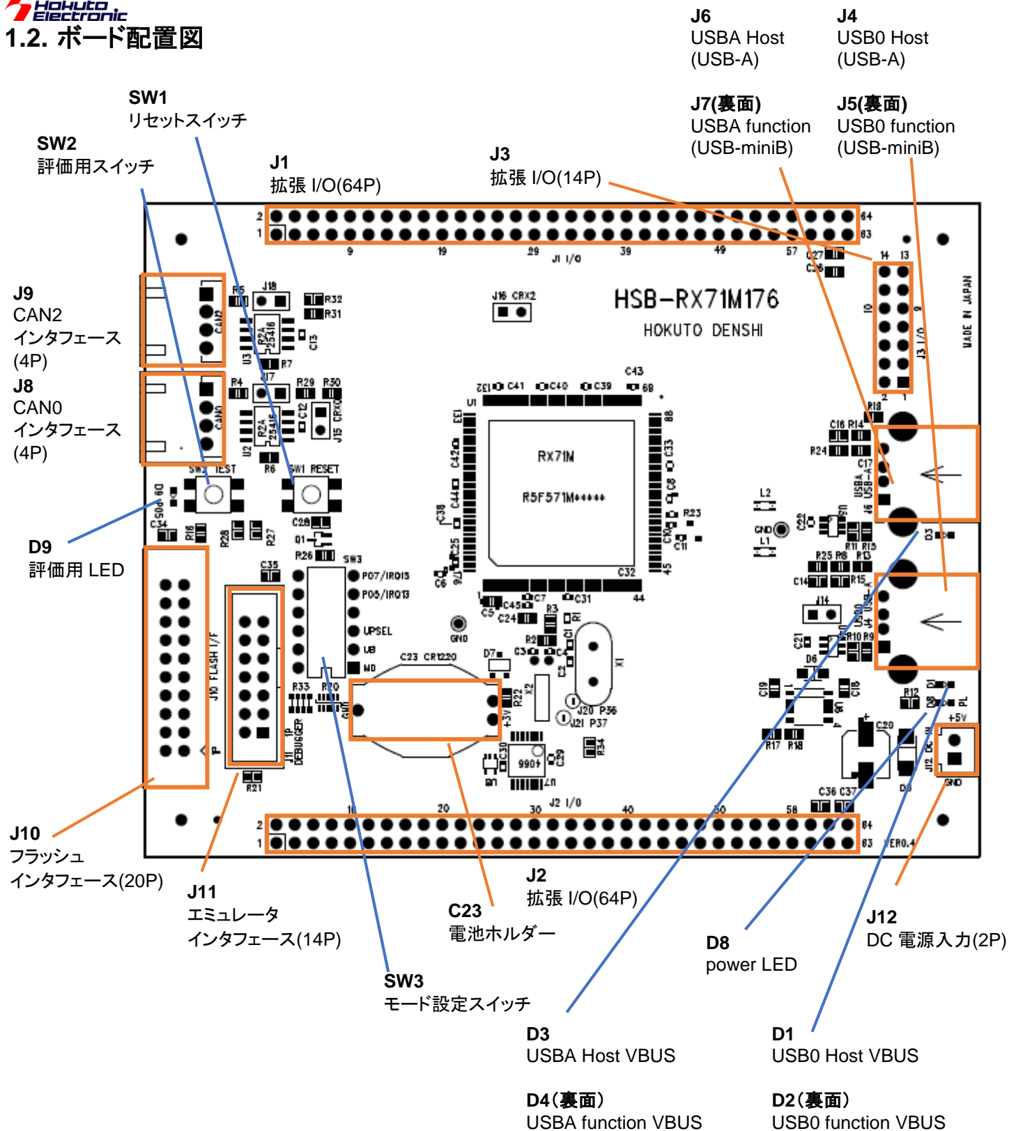
図 1-1 ボード配置図
