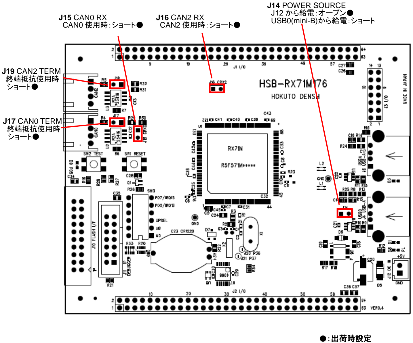
図 1-2 ボード配置図(ジャンパ)
