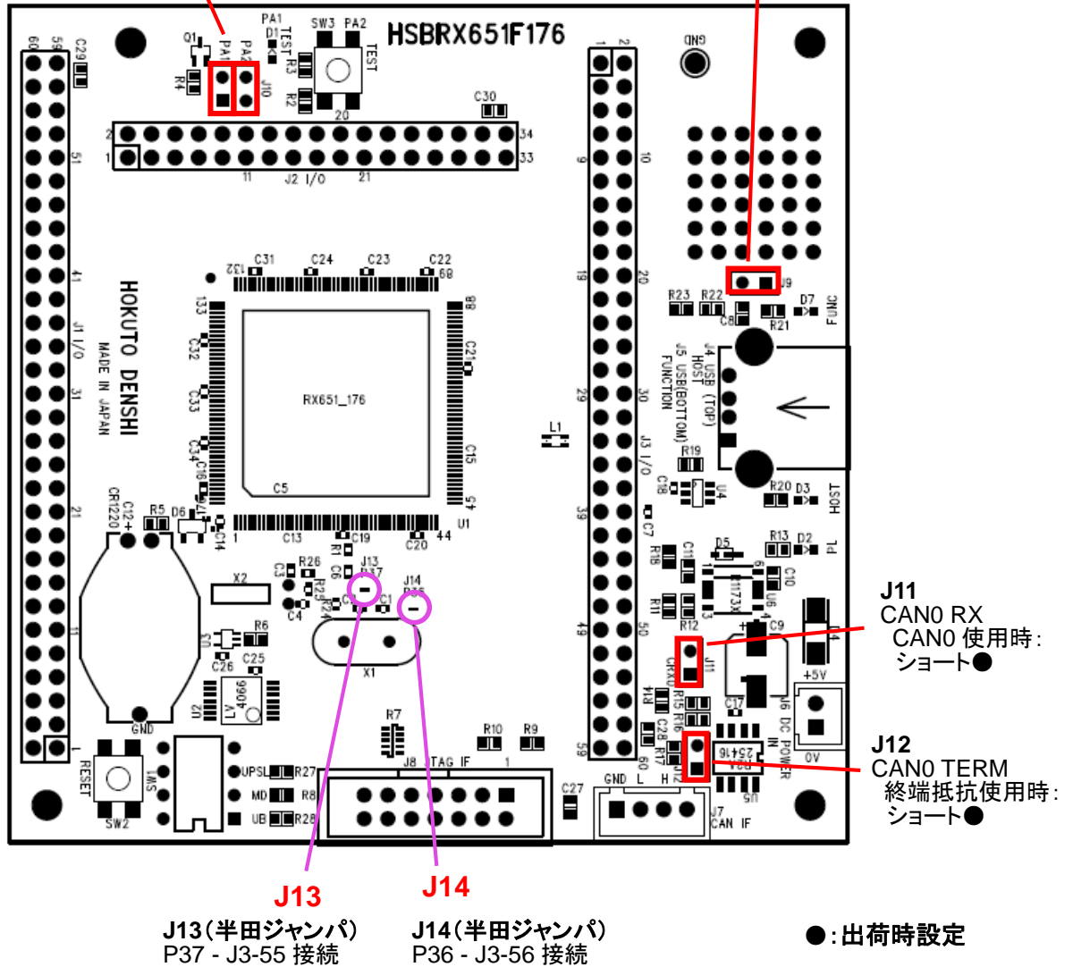
図 1-2 ボード配置図(ジャンパ)
