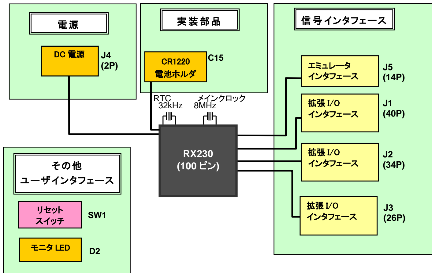
図 1-3 ブロック図
