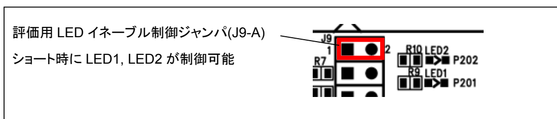
図 2-6 評価用 LED イネーブル制御ジャンパ設定図 (J9-A)
