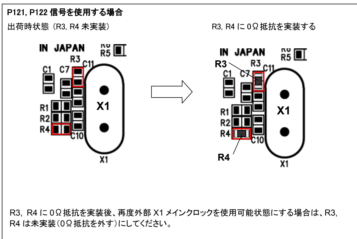
図 2-5 R3, R4 抵抗設定図
