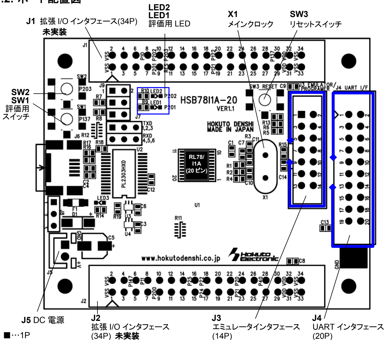
図 1-1 ボード配置図
