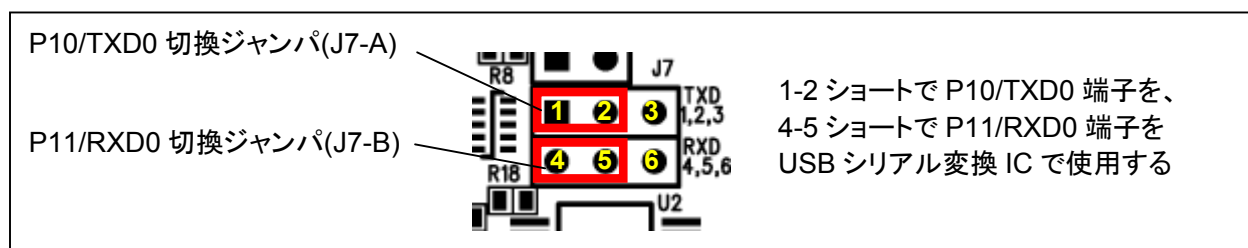
図 2-3 J7 ジャンパ設定図
