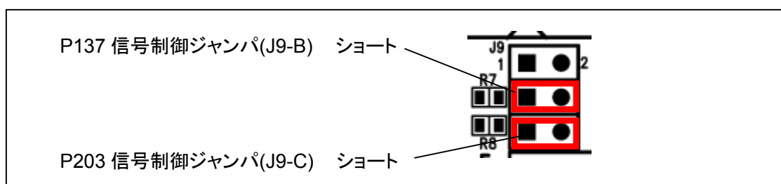
図 2-7 P137, P203 信号制御ジャンパ設定図 (J9-B, J9-C)
