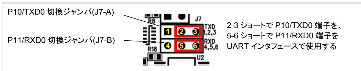
図 2-4 J7 ジャンパ設定図
