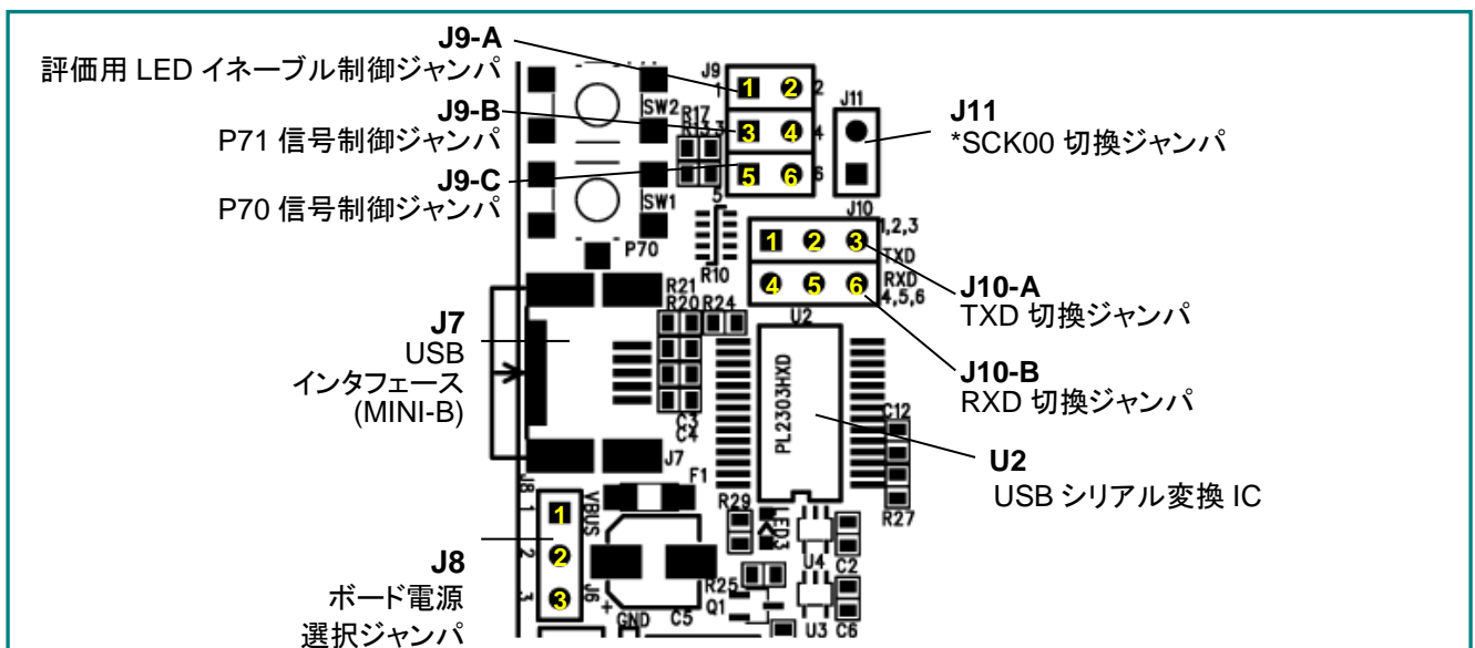
図 1-2 ボード配置補足図
