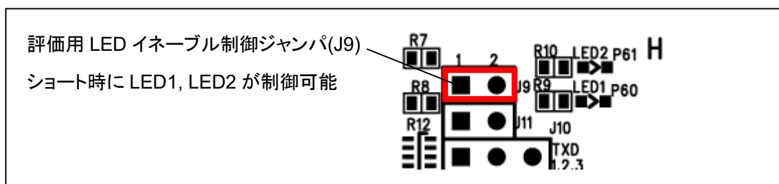
図 2-8 評価用 LED イネーブル制御ジャンパ設定図 (J9)
