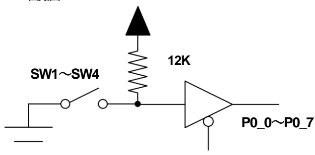
SW 回路図
