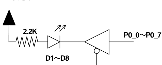
LED 回路図
