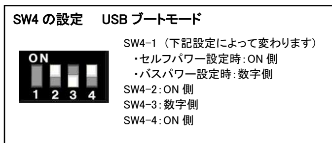
図 3-4 SW4 ジャンパ設定図3
