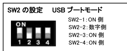
図 5-4 SW2 ジャンパ設定図3
