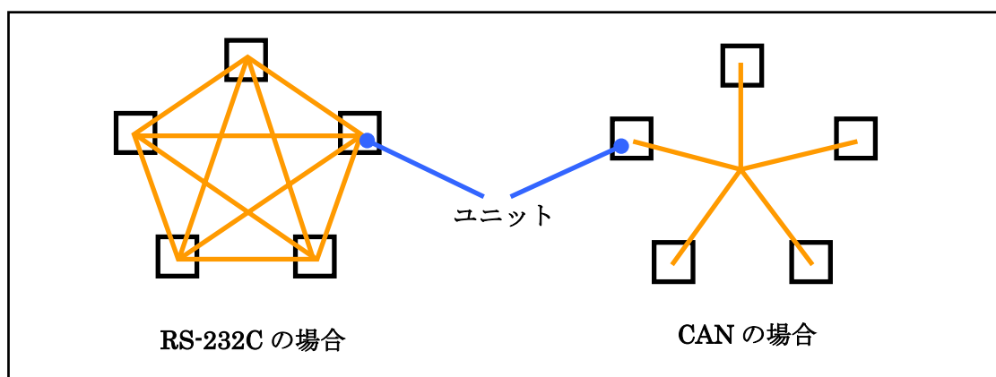
図 1.1 RS232C と CAN のネットワーク接続の比較
